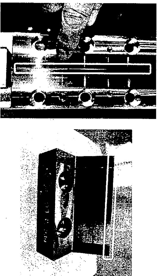
圖 3：安裝在模具設備上的熔噴頭實體 (左) 和熔噴頭模具樣品 (右) 註：白框內即上述細如髮絲的噴絲口。(照片為作者訪談時拍攝)
