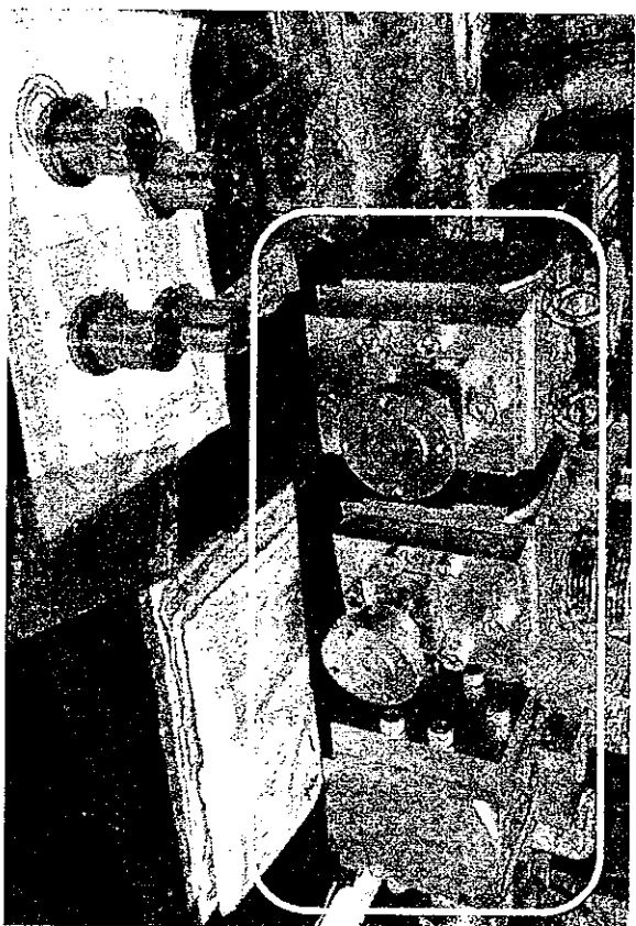
圖 5：控制出料的齒輪泵及其零組件（白框處為齒輪泵本體）
